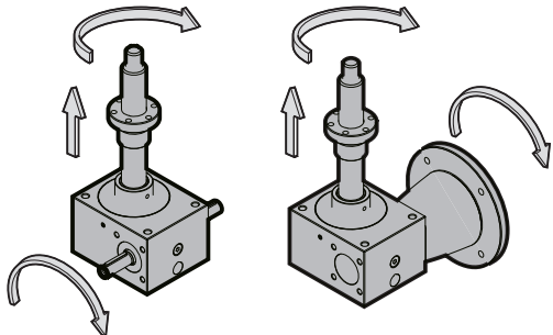
Martinetto Screwjack Hubgetriebe
